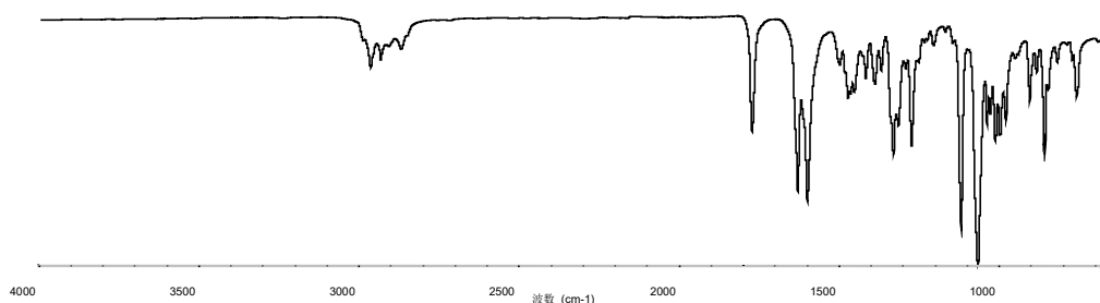
图1 唑啉草酯标样红外光谱图
